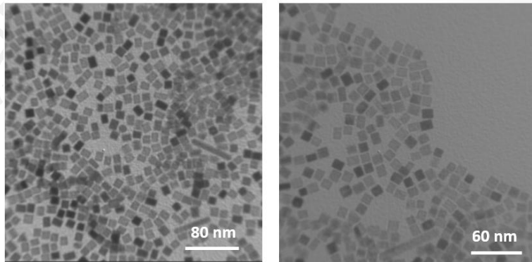
图 1. 11 nm 钯纳米立方体的透射电镜图
