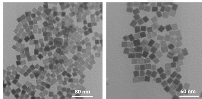
图 1. 17 nm 钯纳米立方体的透射电镜图
